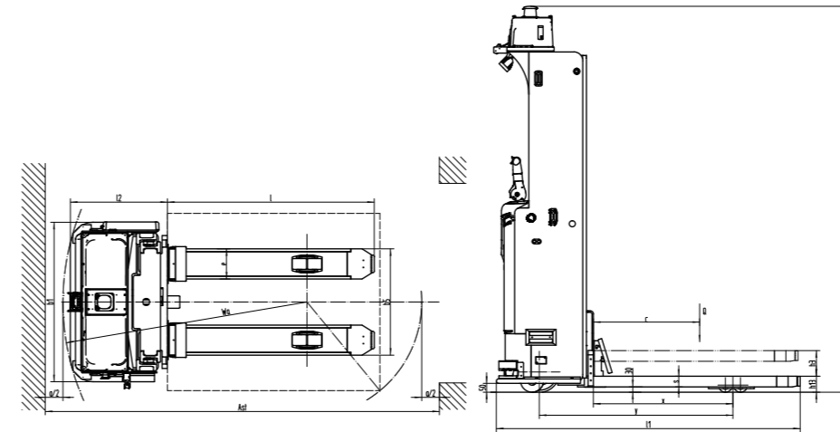
侧视图
