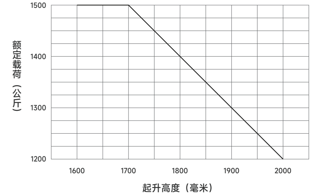
载荷曲线图
